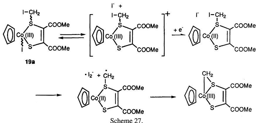
Scheme 27.
