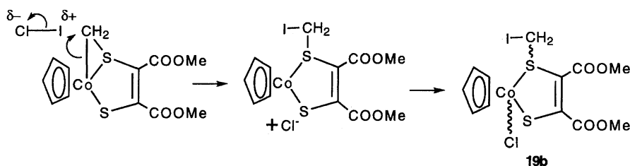
Scheme 26.
